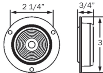
MC52 Reflex Flange
